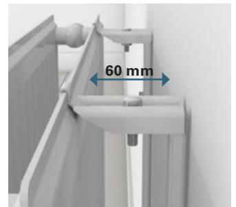
60 mm avstånd mellan vägg och radiator gör det enkelt vid rengöring.
